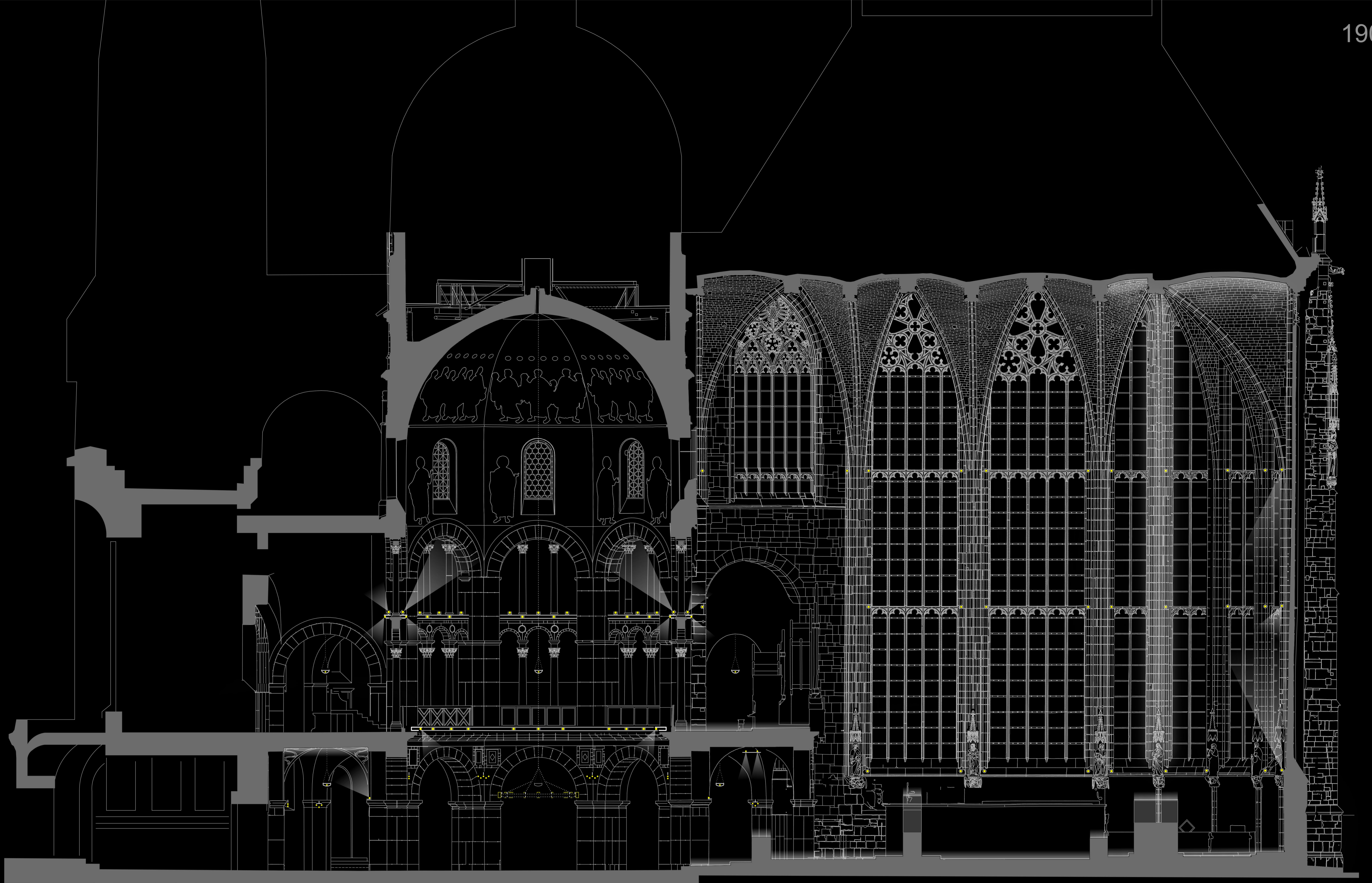
Schnittansicht A.A_Oktogon Chorhalle_M 1: 100
