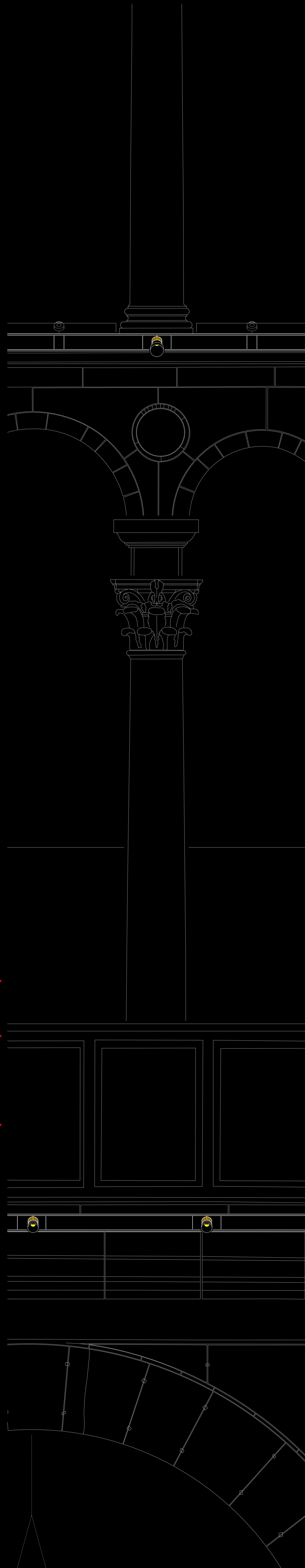
Detail Ausleuchtung_Lichtgesims Ansicht Oktogon_M 1:10
